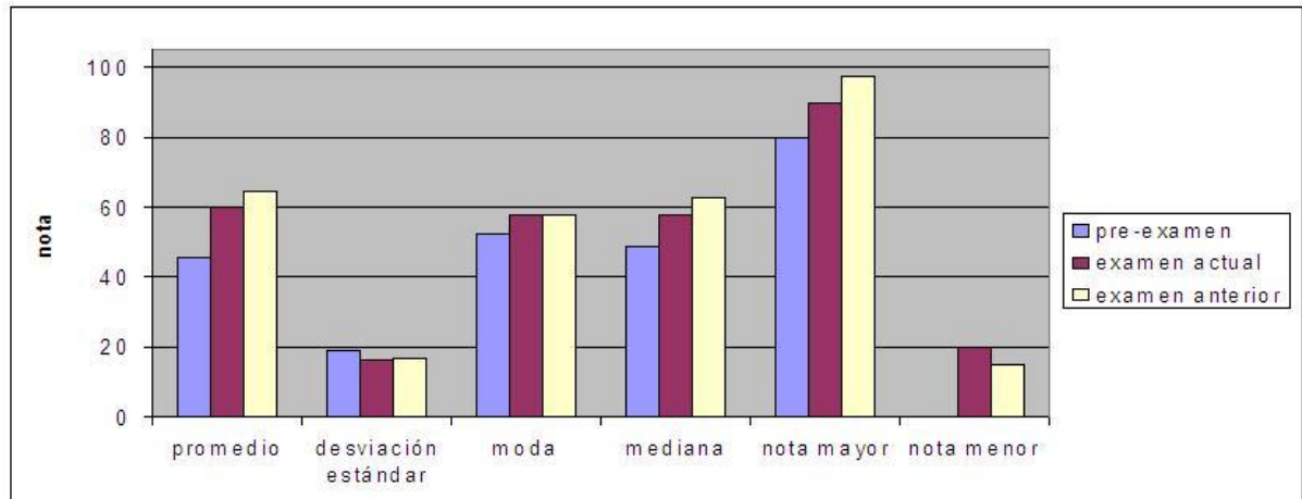
Gráfico 4: Desempeño total del examen
