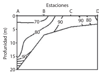
Fig. 6. Variación de la turbidez del agua (JTU) a lo largo de un eje longitudinal esquemático en el Embalse Angostura, Turrialba, Costa Rica.
