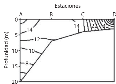
Fig. 8. Variación de la clorofila a ( \text{mg}\cdot\text{m}^{-3} ) a lo largo de un eje longitudinal esquemático en el Embalse Angostura, Turrialba, Costa Rica.
