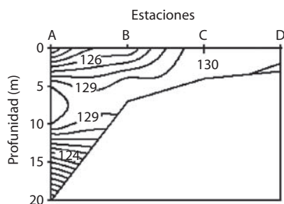
Fig. 5. Variación de la conductividad ( \mu\text{Si-cm}^{-1} ) a lo largo de un eje longitudinal esquemático en el Embalse Angostura, Turrialba, Costa Rica.
