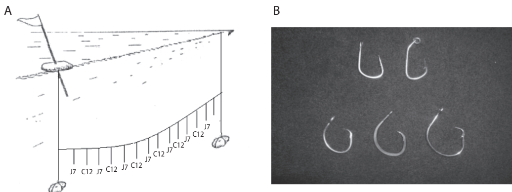
Fig. 1. A. Espinel experimental de fondo utilizado en los monitoreos; B. Anzuelo tradicional (arriba) y anzuelo curvo (abajo). Fig. 1. A. Experimental bottom long-line used in the monitoring; B. traditional hook (above) and circle hook (below).
