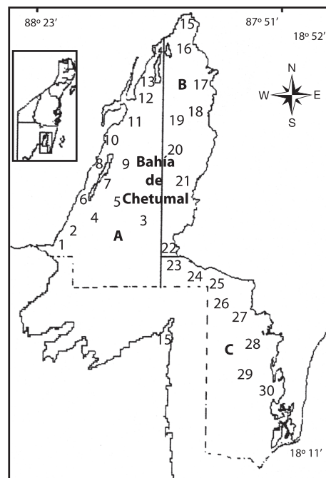
Fig. 1. Ubicación de las 30 estaciones de muestreo en tres sectores de la Bahía de Chetumal. Sector A: 1) Bellavista 2) UQROO 3) Bahía Centro 4) Calderitas 5) Calderitas Exterior 6) Tamalcab Sur 7) Tamalcab Centro 8) Tamalcab Norte 9) Tamalcab-2 Hermanos 10) La Saladora 11) Punta Lagarto 12) La Barra 13) Cayo Venado Sur 14) Cayo Venado-Norte. Sector B: 15) Río Crick 16) Punta Gorda-Cayo Violín 17) Siete Esteros 18) Punta Nicté-Chón 19) La Barra-Punta Nicté-Chón 20) Punta Nicté-Chón-Dos Hermanos 21) Dos Hermanos 22) Punta Flor-Punta Calentura. Sector C: 23) Punta Calentura 24) Cayo Cazón 25) Punta Jazz 26) Punta Mainada-Punta Jazz 27) Punta Mainada 28) Siete Mogotes 29) Mala Noche 30) La Aguada.
