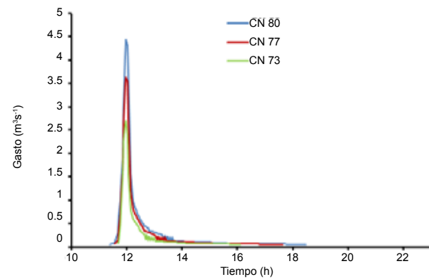
FIGURA 5. Hidrograma en el punto de aforo de la cuenca para un evento de precipitación de 65.2 mm.
