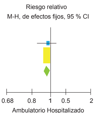
Figura 2 Diagrama de bosque ( forest plot ) de la falla terapéutica del tratamiento ambulatorio frente al tratamiento hospitalizado. Los cuadrados a la izquierda de la línea vertical indican una disminución en el riesgo de desarrollar el fracaso del tratamiento en los pacientes que reciben tratamiento ambulatorio. Las líneas horizontales a través de los cuadrados representan los intervalos de confianza (IC) al 95 %. Los diamantes representan el efecto global del riesgo (RR) del metaanálisis y el correspondiente IC 95 %
