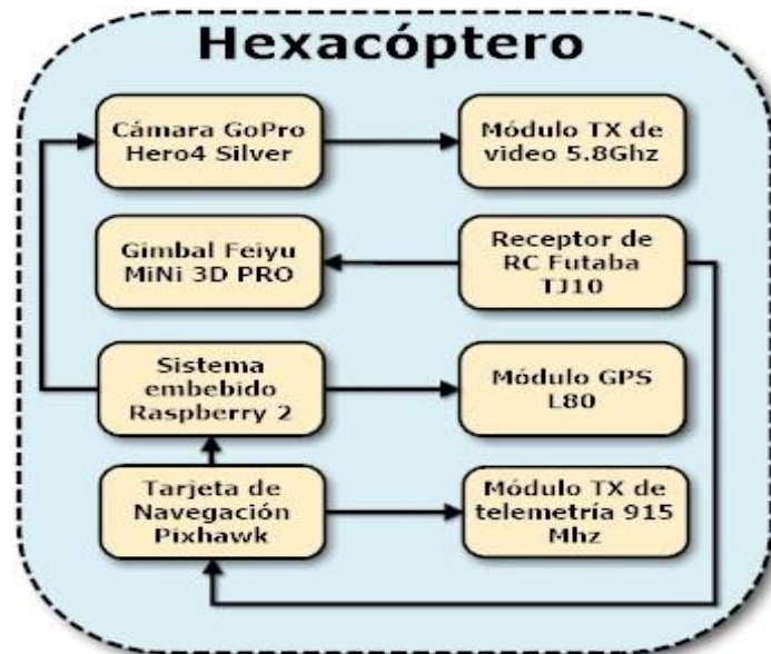
Figura 3. Diagrama a bloques de hardware integrado a hexacóptero.
