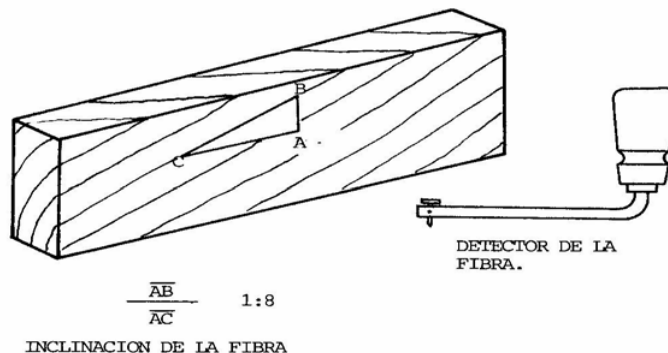
Figura 5. Medición de la inclinación del grano
