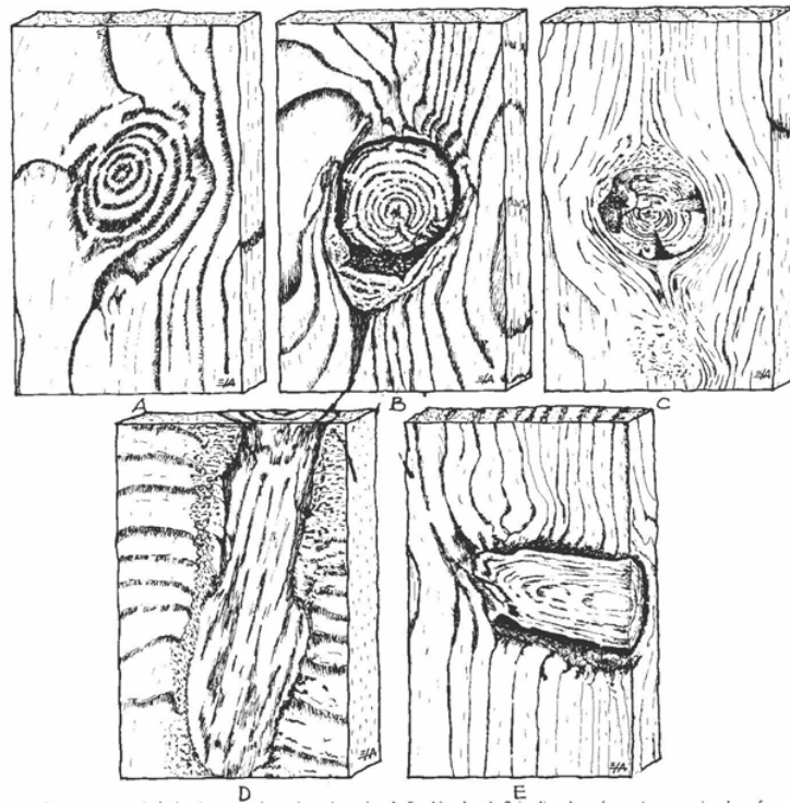
Figura 6. Esquema de los principales tipos de nudos en la madera: (A) nudo fijo, (B) y (C) nudo flojo, (D) nudo en forma de perno, (E) nudo en forma de perno mostrando la porción fija y la floja (Eenique y Robles, 1993)
