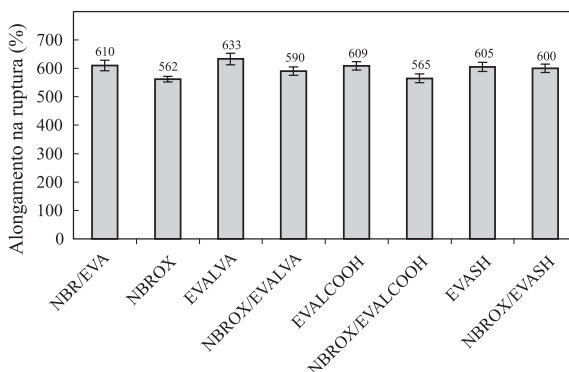
Figura 3. Efeito da natureza do agente de compatibilização no alongamento na ruptura de misturas NBR/EVA
