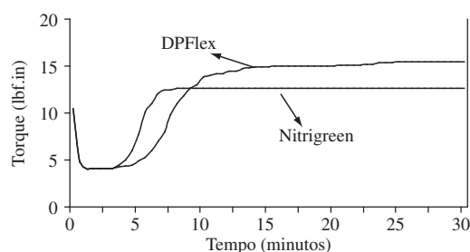
Figura 2. Curvas de torque x tempo obtidas em reômetro de disco oscilatório para borrachas.
