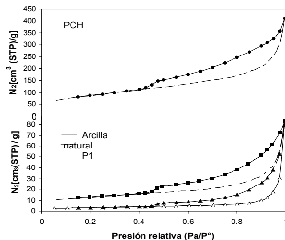
Fig. 6. Isothermas de adsorción-desorción de N_2 (-196°C) de la arcilla natural, la muestra P1 y de la PCH preparada. Símbolos vacíos: adsorción; símbolos llenos: desorción.
