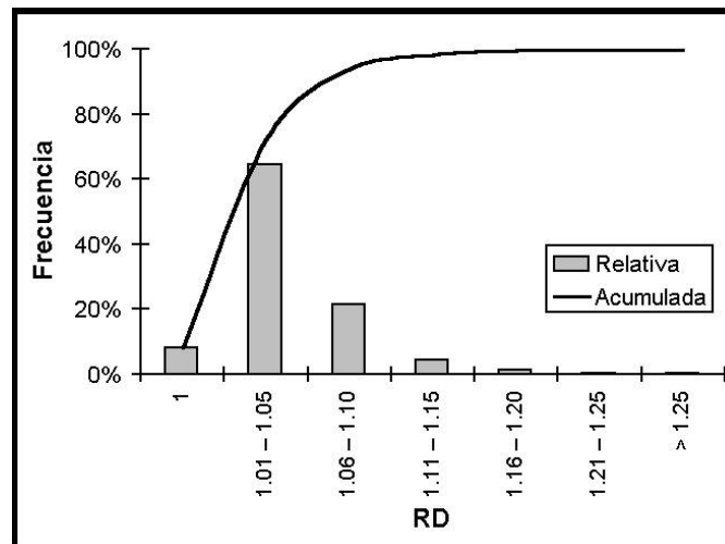
Figura 1. Distribución relativa y relativa acumulada de la razón de diámetros ( RD ) como indicador de la excentricidad de la sección normal.
