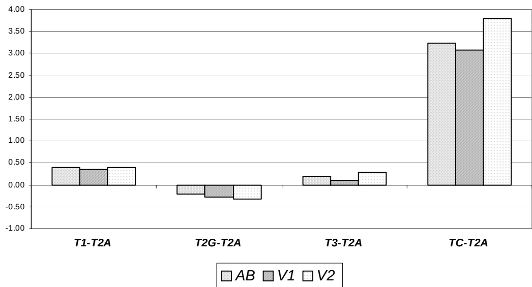
Figura 4. Diferencias en los promedios entre los tratamientos ( T1 , T2G , T3 y TC ) y el tratamiento testigo ( T2A ), para área basal ( AB ) y los volúmenes 1 y 2.
