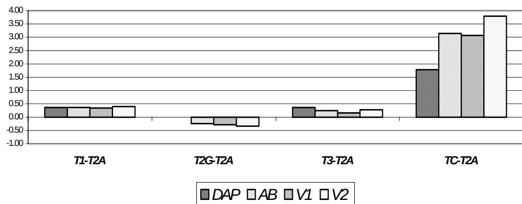
Figura 3. Diferencias en los promedios entre los tratamientos ( T1 , T2G , T3 y TC ) y el tratamiento testigo ( T2A ), para DAP , área basal ( AB ) y V1 y V2 .
