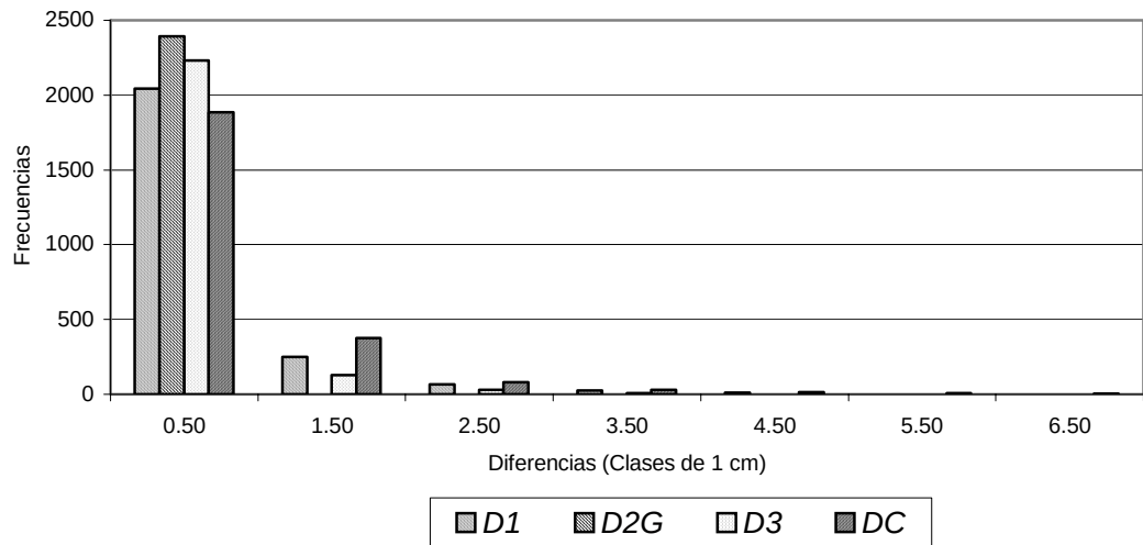
Figura 2. Frecuencias de las diferencias entre el diámetro D2A y los diámetros D1 , D2G , D3 y DC en clases de 1 cm de extensión; valores absolutos.
