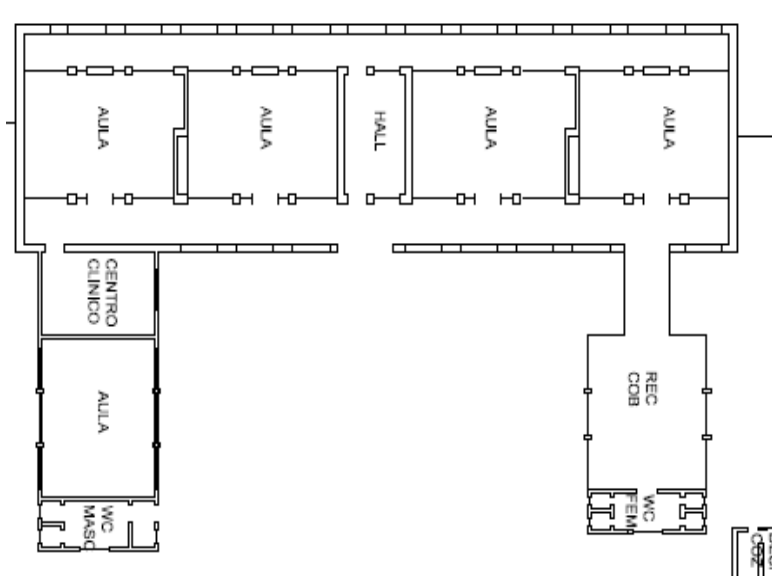
Figura 1: Planta baixa do Jardim de Infância Modelo – Natal, RN (Fonte: SMCE/SEEC/RN)
