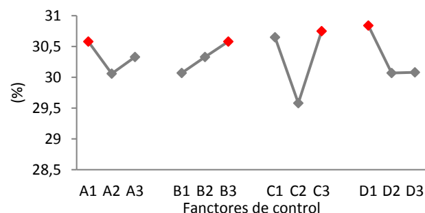
Figura 5. Efecto promedio de la relación señal/ruido sobre el valor medio del rendimiento de pulpa de celulosa de la especie A. salmiana con el método de pulpeo Organosolv (CH 3 COOH). Fuente: Elaboración propia
