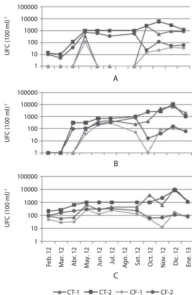
Fig. 2. Cantidad de coliformes totales y de coliformes fecales en los ríos Chitá (a), Ixconá-Sis (b) y Sacobá (c), en unidades formadoras por cada 100 ml. Notas: CT-1= coliformes totales en la cabecera, CT-2 = coliformes totales en la desembocadura, CF-1 = coliformes fecales en la cabecera, CF-2 = coliformes fecales en la desembocadura.
