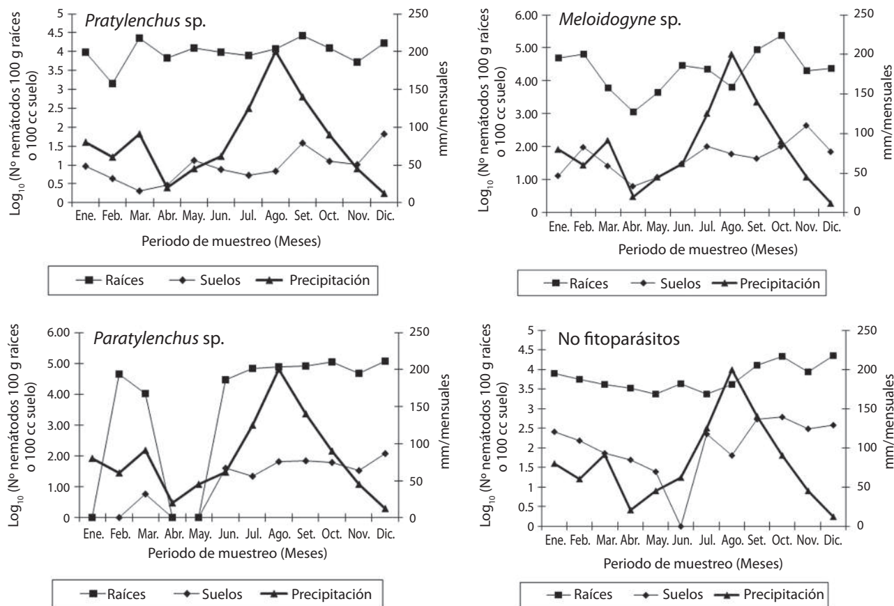
Fig. 2. Fluctuación en la población de nematodos de los géneros Pratylenchus sp., Meloidogyne sp., Paratylenchus sp. y no fitoparásitos presente en muestras de raíces y de suelo en el pasto Ratana. Ciudad Quesada, San Carlos, Alajuela, Costa Rica, 2006.
