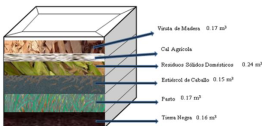
Figura 2. Composición y Estructura Pila 2 y Pila Réplica 2' (ROD+P+M) Residuos Orgánicos + Pasto + Madera Fuente: Autor
