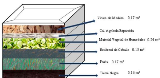
Figura 1. Composición y Estructura Pila 1 y Pila Réplica 1' (MV+P+M) Material Vegetal + Pasto + Madera Fuente: Autor
