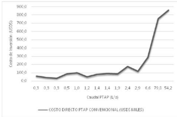
Figura 1. Costo de inversión y caudal de diseño para PTAP Convencional
