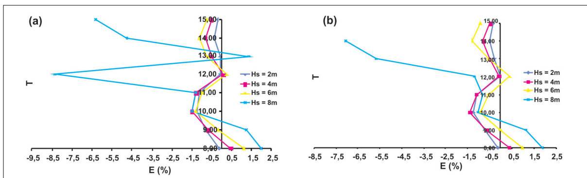
Figura 10 - Influência do T_p para o FPSO na condição FAR CROSS com conexão no turrete. (a) CD = 0,9; (b) CD = 1,2.
