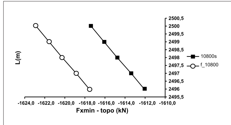
Figura 6 - Envolvória de força mínima para 1 simulação.
