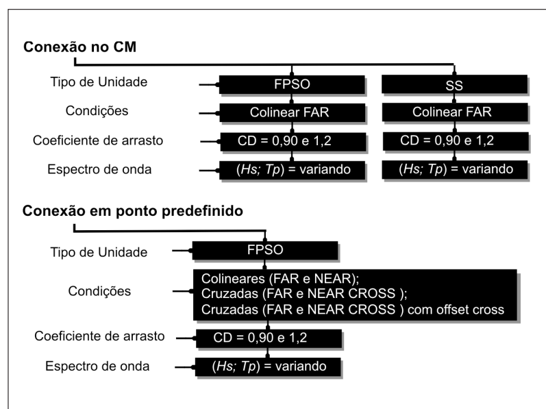
Figura 1 - Casos de carregamento utilizados para determinação do caso crítico.
