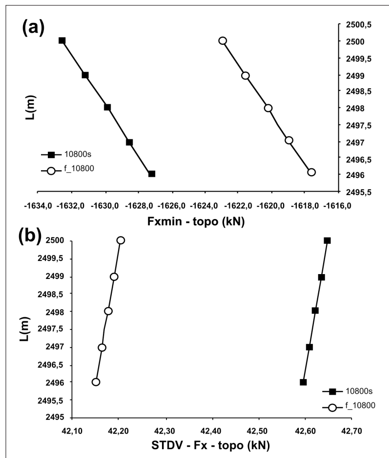
Figura 5 - Envoltórias de força mínima e desvio-padrão médio no topo para 10 simulações. (a) força mínima média; (b) desvio-padrão médio.
