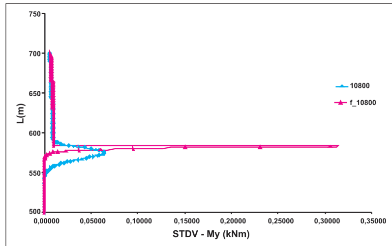
Figura 8 - Curvas de desvio-padrão de momentos no TDP.
