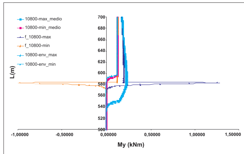
Figura 7 - Curvas de momentos no TDP.
