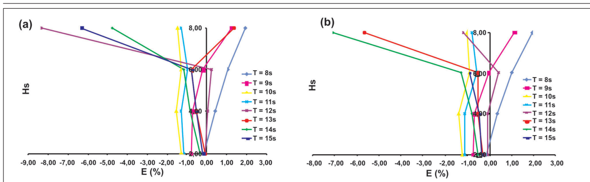
Figura 9 - Influência do H_s para o FPSO na condição FAR CROSS com conexão no turrete. (a) CD = 0,9; (b) CD = 1,2.
