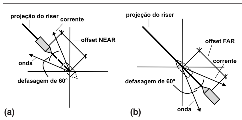
Figura 3 - Casos de análise não colineares, offsets NEAR e FAR. (a) caso NEAR CROSS; (b) caso FAR CROSS.
