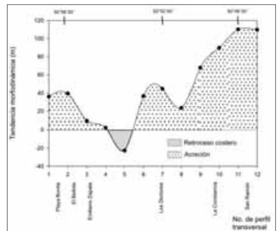
Figura 7. Variaciones de la línea de costa de la hoja E15B71 (Villa Vicente Guerrero), a escala 1:50 000, durante el período 1972-1995. Como contraste con el resto de la zona costera tabasqueña, en este sector se desarrolla un intenso proceso de acreción, con valores hasta de +8 m/año y +10 m/año.
