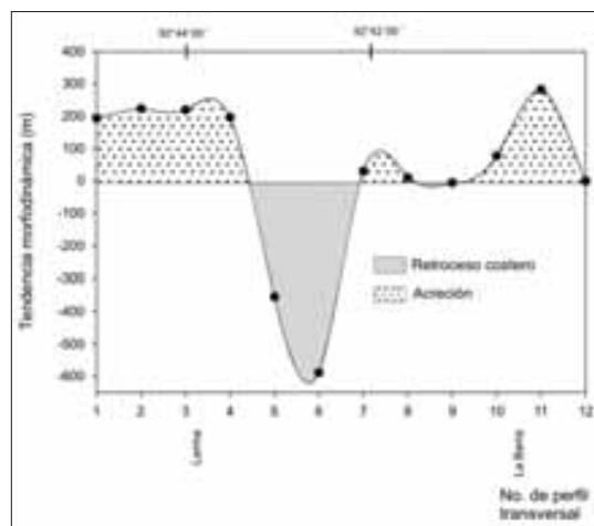
Figura 8. Variaciones de la línea de costa de la hoja E15B61 (Felipe Carrillo Puerto), a escala 1:50 000, durante el período 1972-1995. En este sector se conjugó el proceso de acreción (localidades de Lerma, con +9.6 m/año, y de La Barra, con +12.3 m/año) con el de retroceso intenso, el más notable de todo el estado, en las inmediaciones de la desembocadura del río Usumacinta, con un gradiente de -25 m/año, durante un intervalo de 23 años.
