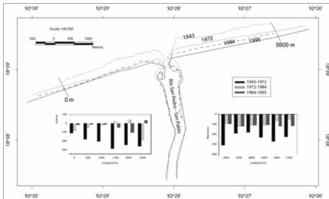
Figura 2. Retroceso de la costa en el frente deltaico del río San Pedro y San Pablo, entre los periodos 1943-1972, 1972-1984 y 1984-1995.
