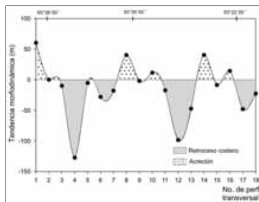
Figura 5. Variaciones de la línea de costa de la hoja E15A78 (Cocohital), a escala 1:50 000, durante el período 1984-1995. Obsérvense los gradientes de retroceso costero de -11.5 m, en la localidad de El Alacrán, y de -9 m/año, en Barra de Tupilco.
