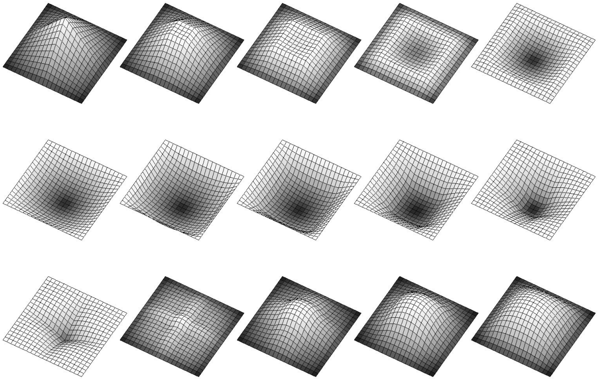
FIGURA 3. De izquierda a derecha, de arriba hacia abajo, se muestra la evolución temporal de la membrana cuadrada con la configuración inicial en forma de la función (15); cada toma presentada está separada por intervalos de tiempos iguales y de valor \Delta T = T_{1,1}/14 .
