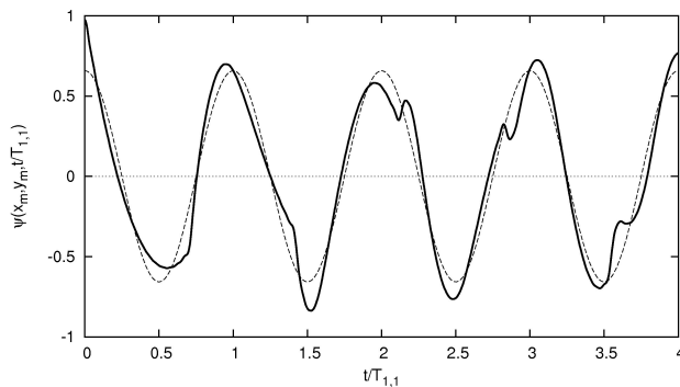
FIGURA 4. Movimiento en el centro de la membrana cuadrada respecto al tiempo. Se observa hasta un tiempo igual a t = 4T_{1,1} . También se muestra el comportamiento del modo de frecuencia más bajo en el mismo punto de la membrana (línea punteada).
