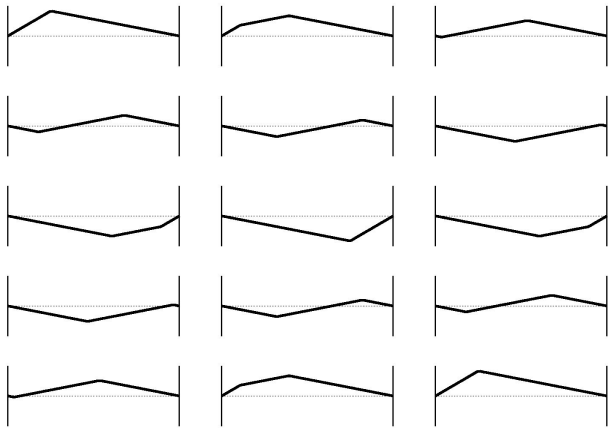
FIGURA 2. De izquierda a derecha, de arriba hacia abajo, se muestra la evolución temporal de la cuerda con la configuración inicial en forma de triángulo con vértice a L/4 ; cada toma presentada está separada por intervalos de tiempos iguales y de valor \Delta T = T_1/14 .
