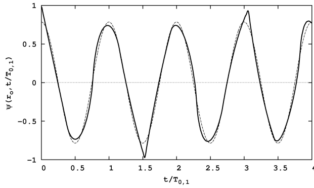
FIGURA 6. Movimiento en el centro de la membrana circular respecto al tiempo. Se observa hasta un tiempo igual a t=4T_{0,1} . También se muestra el comportamiento del modo de frecuencia más bajo en el mismo punto de la membrana (línea punteada).
