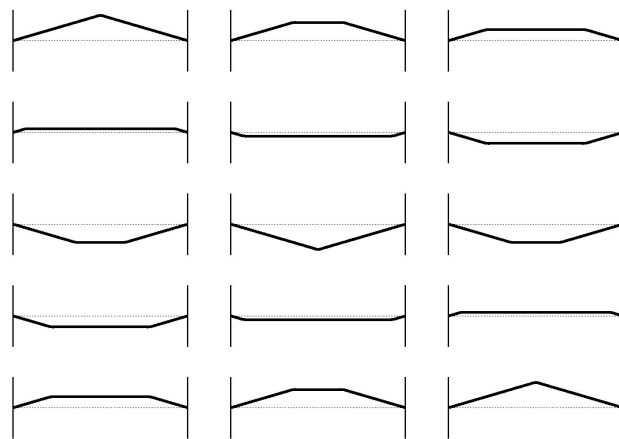
FIGURA 1. De izquierda a derecha, de arriba hacia abajo, se muestra la evolución temporal de la cuerda con la configuración inicial en forma de triángulo; cada toma presentada está separada por intervalos de tiempos iguales y de valor \Delta T = T_1/14 .
