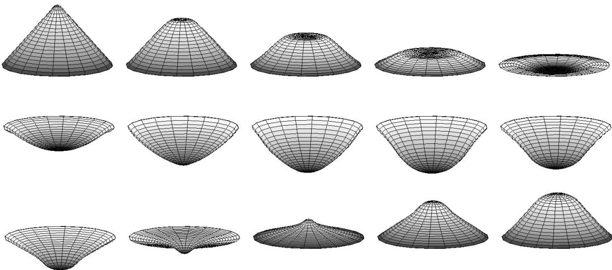
FIGURA 5. De izquierda a derecha, de arriba hacia abajo, se muestra la evolución temporal de la membrana circular con la configuración inicial en forma de cono circular; cada toma presentada está separada por intervalos de tiempos iguales y de valor \Delta T = T_{0,1}/14 .
