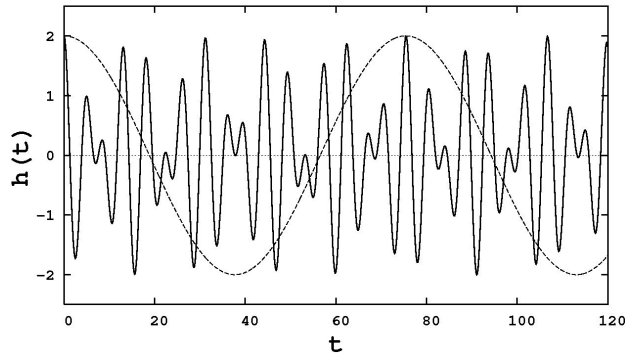
FIGURA 7. La función h(t) = \cos(t) + \cos(\sqrt{2}t) (línea sólida) no es periódica, pero sí es cuasi-periódica. En este caso se muestra uno de los cuasi-periodos mediante una función armónica con periodo T=24\pi (Línea punteada).
