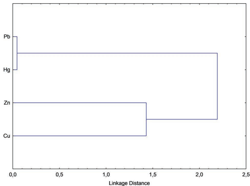
Figura 2. Dendrograma de agrupación jerárquica de los metales pesados.
