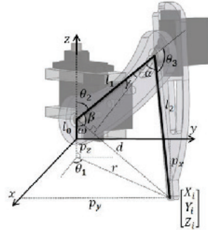
Fig. 4. Parámetros cinemática inversa. Fuente: Autores del proyecto
