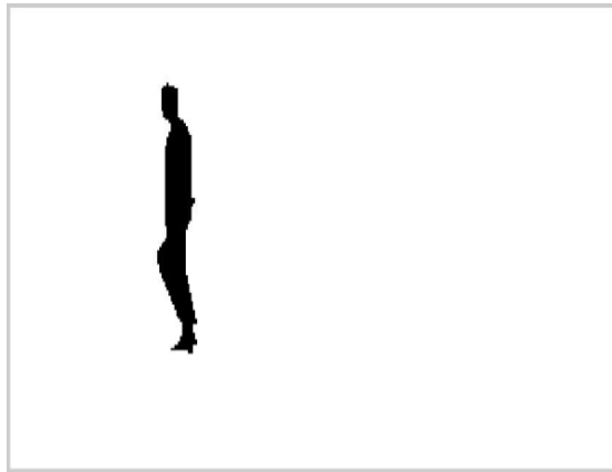
Fig. 4. Segmentación manual
