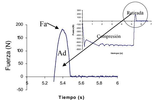
Fig. 2. Curva modelo de adhesividad.
