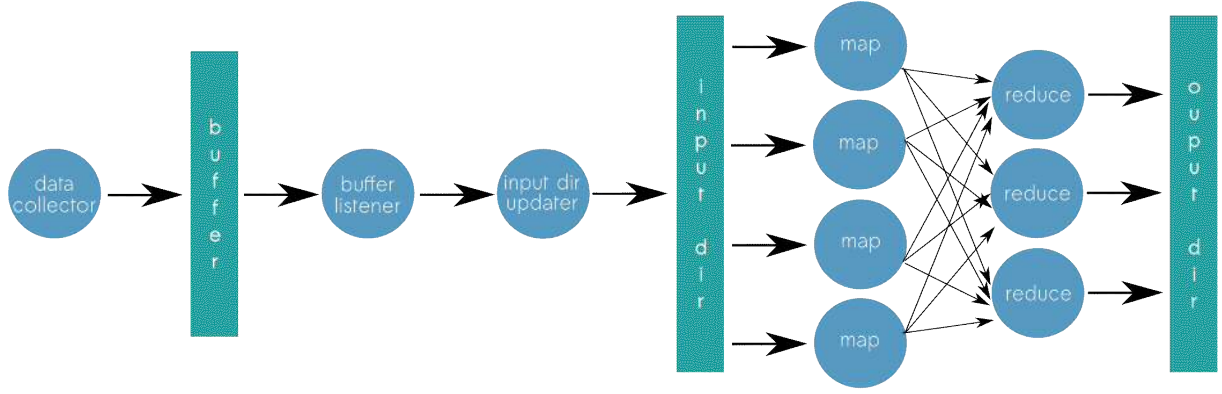
Figure 1: DAG
