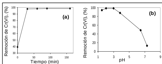
Figura 3. a) Determinación del tiempo de equilibrio para la adsorción de Cr(VI) sobre alúmina. b) Efecto del pH inicial, con un tiempo de contacto de 1 hora. En ambos experimentos se utilizaron los siguientes parámetros: concentración inicial de Cr(VI) = 10 \text{ mg L}^{-1} , 0.25 \text{ g} de alúmina, volumen de solución = 25 \text{ mL} , \text{pH} = 2 y agitación = 150 \text{ rpm} .
