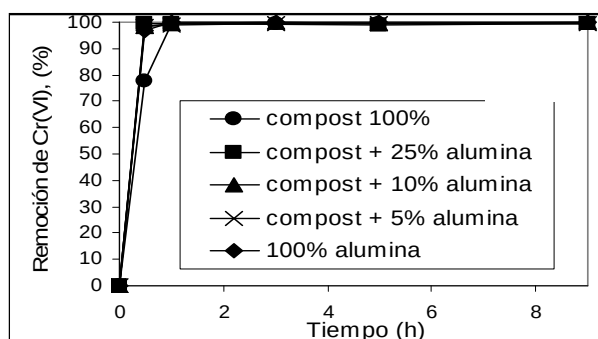
Figura 7. Efecto de la adición de alúmina al compost 1 para la eliminación de Cr(VI) (concentración inicial de Cr(VI) = 3,0 mg L -1 ). Condiciones experimentales: 2,5 g de compost, 100 mL de solución, pH = 2,5 y 150 rpm.
