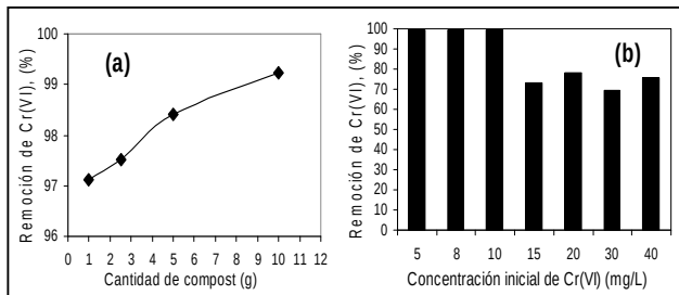
Figura 6. a) Efecto de la cantidad de compost 1 en la eliminación de Cr(VI), concentración inicial de Cr(VI) = 5 \text{ mg L}^{-1} . b) Efecto de la concentración inicial de Cr(VI), 2.5 g de compost 1. Las condiciones experimentales fueron iguales en ambos ensayos: 100 mL de solución, pH = 2.5, 150 rpm, tiempo = 3h.
