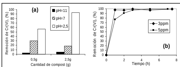
Figura 5. a) Efecto de pH en la eliminación de Cr(VI) empleando dos cantidades de compost 1, con una concentración inicial de Cr(VI) = 5 \text{ mg L}^{-1} . b) Determinación del tiempo de equilibrio para la adsorción de Cr(VI) sobre el compost 1, empleando concentraciones iniciales de Cr(VI) de 3 \text{ mg L}^{-1} y 5 \text{ mg L}^{-1} , pH = 2,5 y 2,5 g de compost. En ambos experimentos se utilizaron 100 mL de solución y agitación a 150 rpm.
