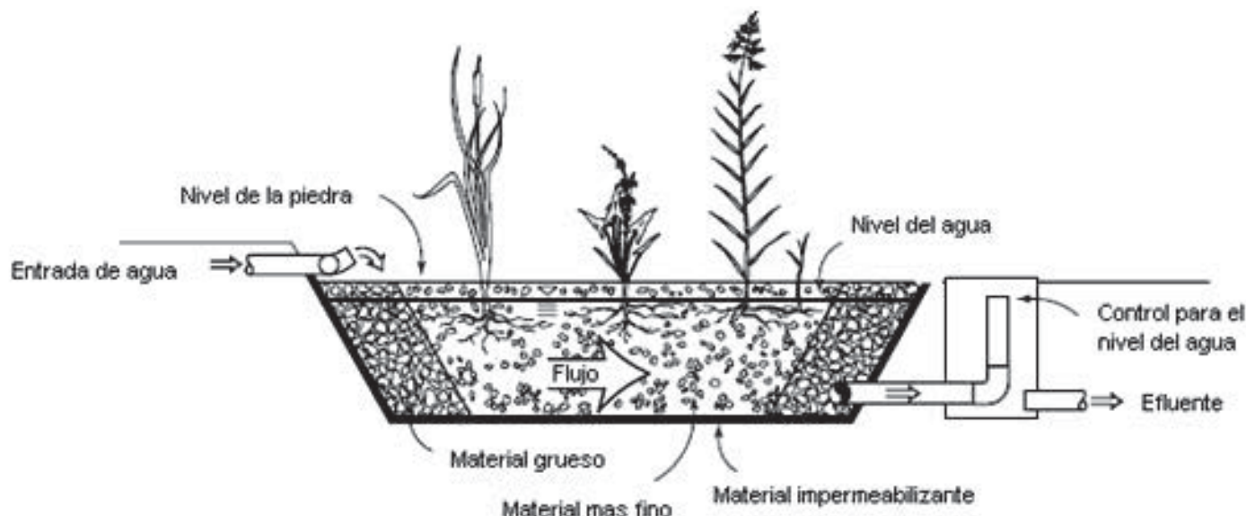
Figura 1. Esquema típico de un humedal artificial para el tratamiento de aguas residuales.
