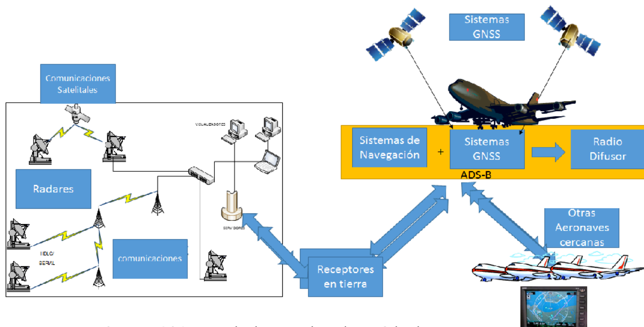
Figura 6. Esquema Sistema ADS-B integrado al sistema de vigilancia Colombiano.
