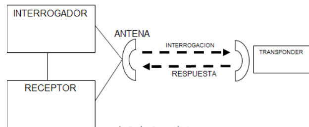
b. Radar Secundario
