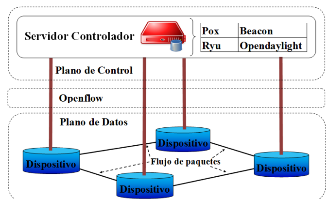
Figura 2. Plano de datos y control con el servidor controlador
