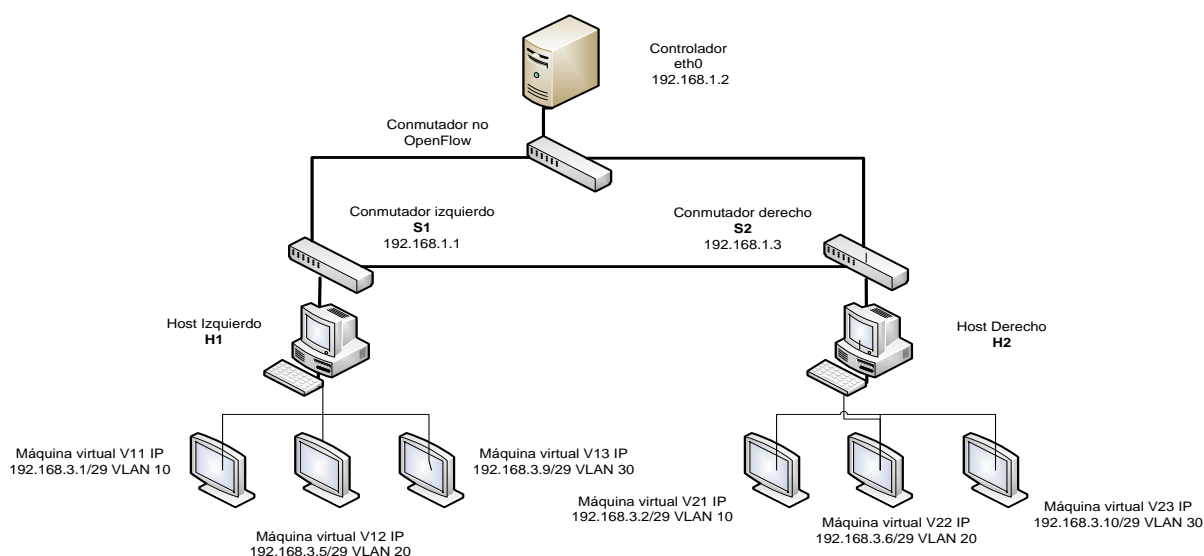
Figura 6. Diagrama de topología para la implementación del prototipo básico
