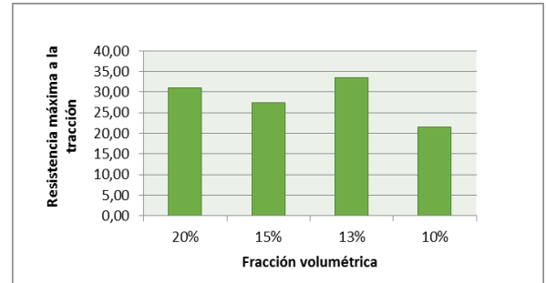
Figura 3. Resistencia a la tracción vs. fracción volumétrica porcentual de fibra de 10mm dispersada aleatoriamente.
