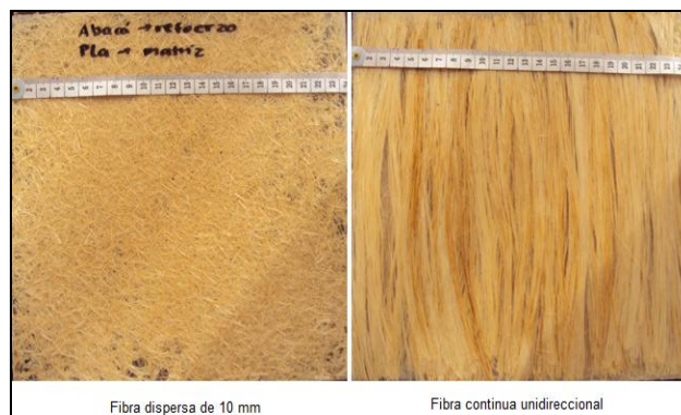
Figura 8. Láminas de material compuesto de matriz de PLA reforzada con fibra natural (Dimensiones de las láminas 239 x 239 mm).
