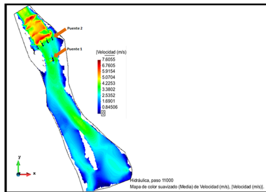
Figura 5: Velocidades a lo largo de la Quebrada La Guardia para el instante de tiempo donde se produce el caudal pico.
