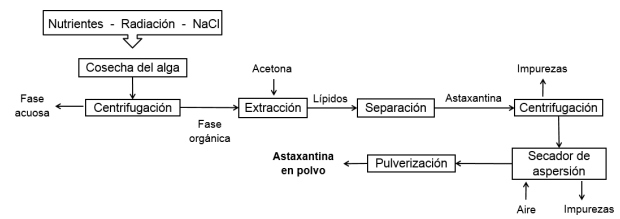
Figura 3: Esquema propuesto del proceso tecnológico para la extracción de astaxantina a partir de una cepa Dunaliella salina .
