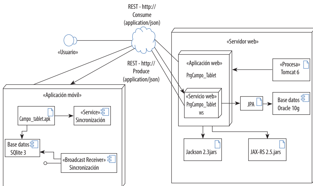
Figura 5. Arquitectura detallada del sistema de computación móvil.
