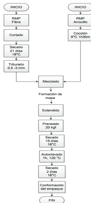
Figura 1. Diagrama de flujo de la elaboración de empaques secundarios ecológicos
