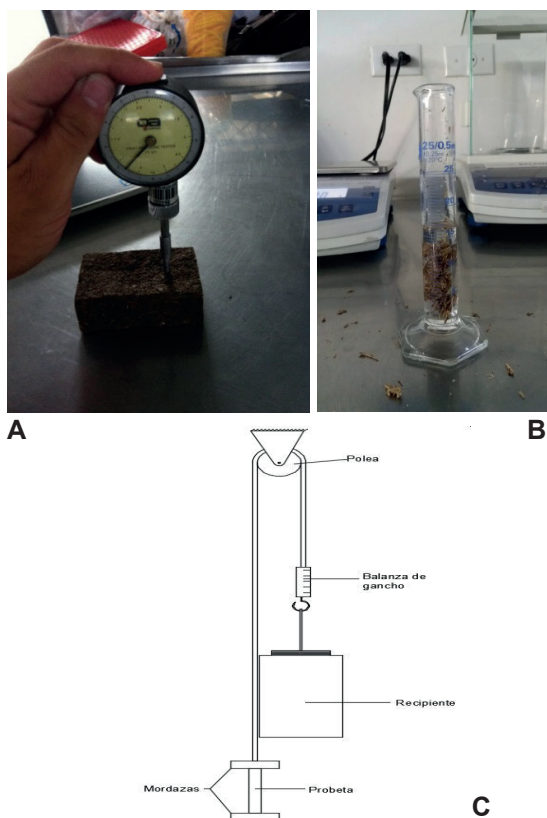
Figura 2. Evaluaciones mecánicas del empaque secundario: 2A. Medición de dureza; 2B. Medición de densidad; 2C. Esquema de equipo para medición de tracción
