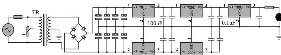
Figura 4: Esquema del circuito de la fuente de alimentación del teslámetro.
