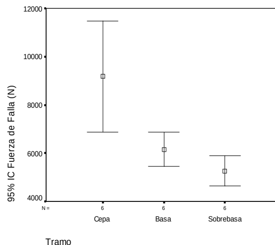
Figura 6. Fuerza de Falla Promedio por Tramo de la Guadua
