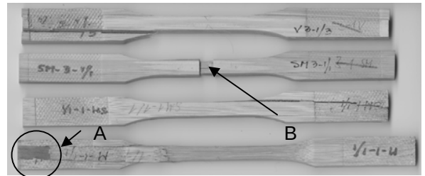
Figura 10. Probetas fracturadas a tensión, pero con desplazamiento de sección A y desplazamiento en garganta B.
