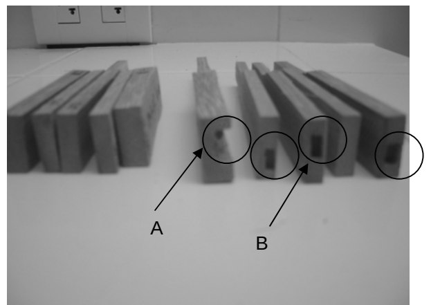
Figura 11. Probetas fracturadas a tensión, mostrando el área de deslizamiento por cizalladura, equivalente al área de la garganta.
