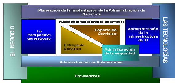
Figura 2. Estructura ITIL
