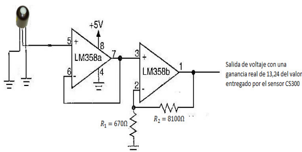
Fig.4. Circuito de acople del sensor CS300 Fuente: Elaboración Grupo GRINDES
