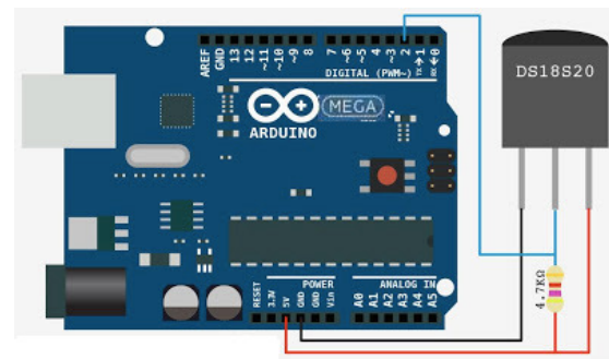
Fig.1. Esquemático acople sensor de temperatura DS18B20 Fuente: Elaboración Grupo GRINDES
