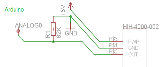
Fig.2. Esquemático acople sensor de humedad HIH-4000-002. Fuente: Elaboración Grupo GRINDES
