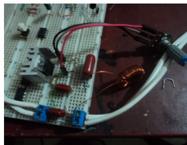
Figura. 9. Primera implementación del circuito
