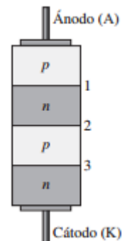
Figura. 3. Diodo de 4 capas [8]
