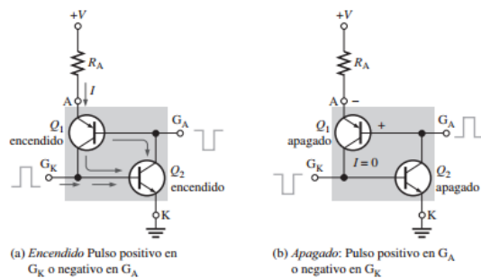
Figura. 5. Operación de un SCS [8]
