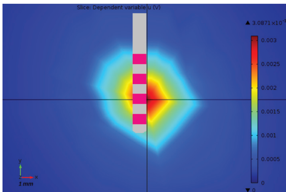
Figura 6. Superficie de activación en el plano XY del modelo anisotrópico Subtalámico para una estimulación constante de corriente de 40 \mu A . El valor máximo de activación de voltaje alcanza 3.15 mV.
