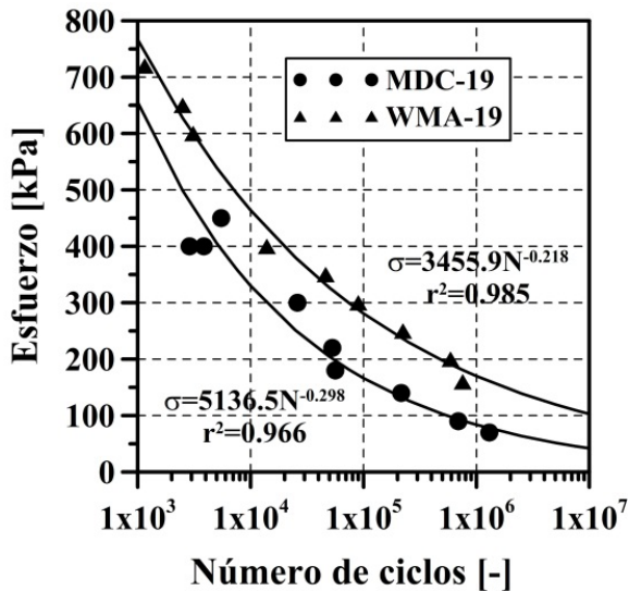
Figura 4. Resistencia a fatiga
