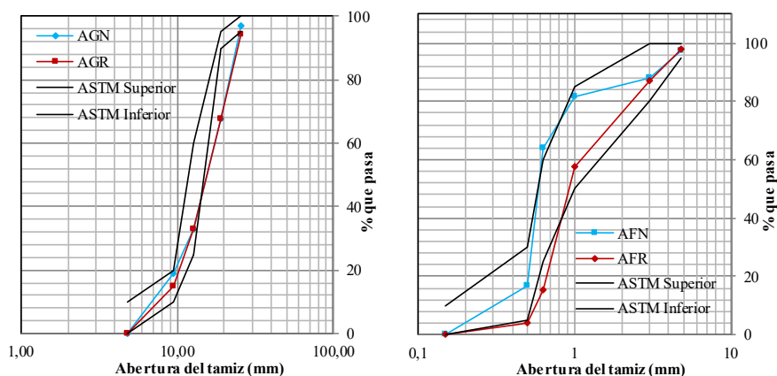
Figura 5. Granulometría de los áridos utilizados en la investigación. 5a) áridos gruesos y 5b) áridos finos.
