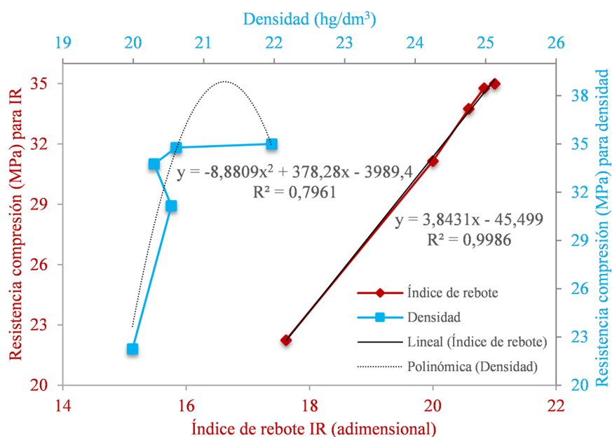
Figura 8. Correlación de resistencia a la compresión y el índice de rebote.
