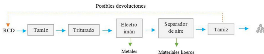
Figura 1. Proceso de reciclaje de los áridos reciclados.
