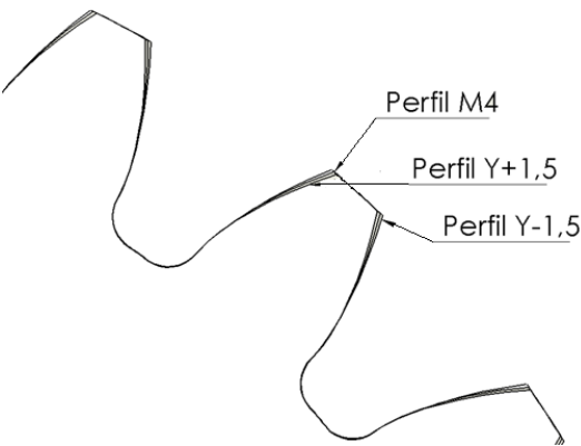
Figura 7. Comparación de la forma de los perfiles M4, Y +1,5 , Y -1,5 por superposición.
