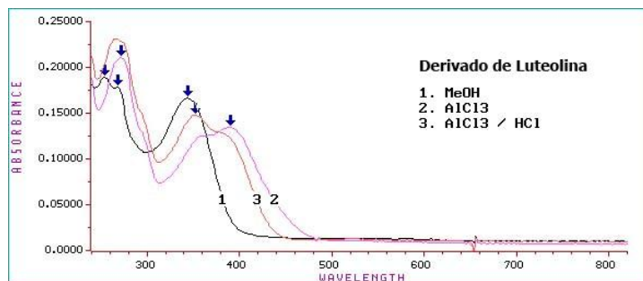
Figura 2: Espectros UV-visible para la flavona derivada de Luteolina. Se muestran los desplazamientos para el reactivo de AlCl 3 y AlCl 3 /HCl.
