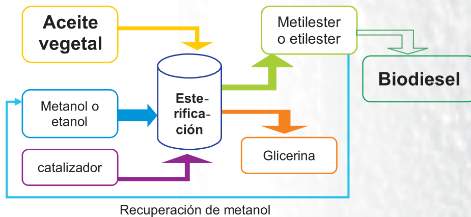
Figura 5. Proceso detallado de producción de biodiesel utilizado en el proyecto.
