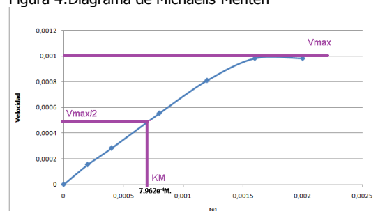
Figura 4:Diagrama de Michaelis-Menten
