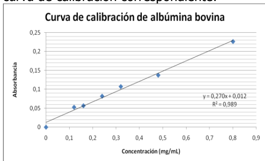
Figura 1: Curva de calibración albúmina bovina para la cuantificación
