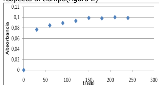
Figura 2: Variación de la absorbancia respecto al tiempo.
