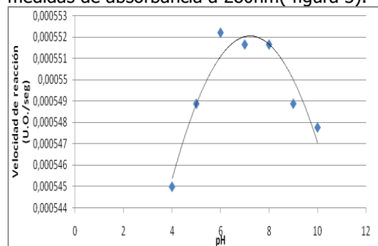
Figura 3: Dependencia de la actividad enzimática de la bromelina respecto del pH.
