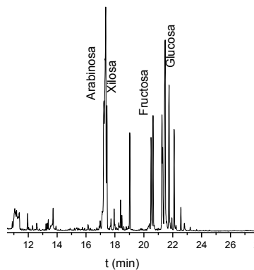
Figura 9. Cromatograma de Hidrolizado BP.
