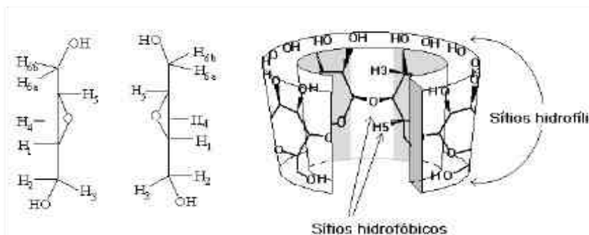
Figura 6. Representación esquemática de las posiciones de los átomos de hidrógeno y O-glicosídicos en la cavidad de la ciclodextrina.
