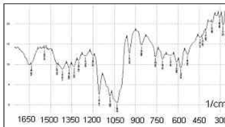
Figura 1. Espectro de absorción en la región infrarroja (1700 - 250 \text{cm}^{-1} ) para la beta ciclodextrina
