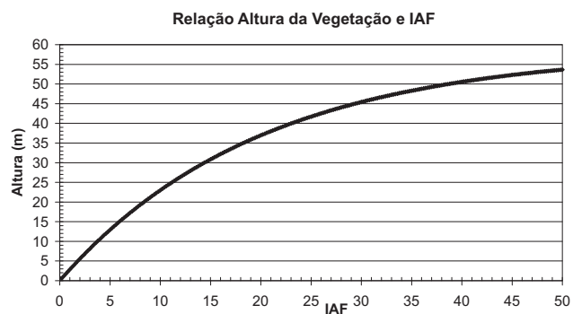
Figura 2. Relação empírica proposta por KELLIHER et al. (1993) entre a altura da vegetação e o IAF.
