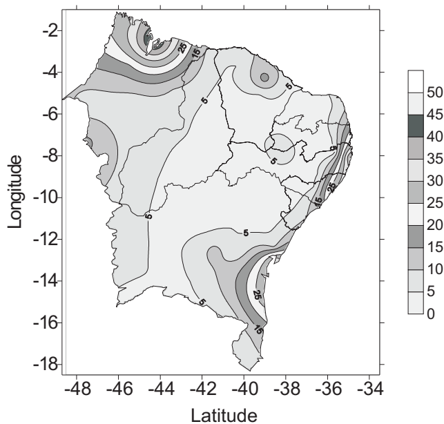
Figura 3. Altura da vegetação potencial em metros para o NEB estimada pelo modelo REY (1999).
