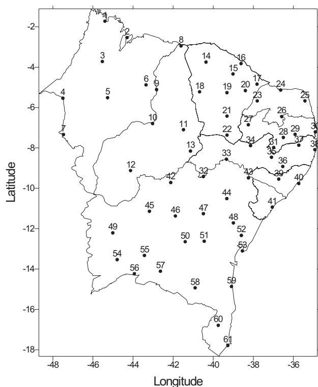
Figura 1. Distribuição espacial das estações climatológicas do NEB usadas no presente trabalho, os números são códigos de cada localidade listados na Tabela 1.
