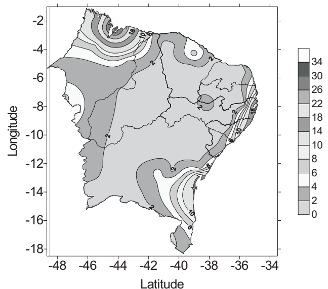
Figura 4. IAF da vegetação potencial para o NEB estimado pelo modelo REY (1999).
